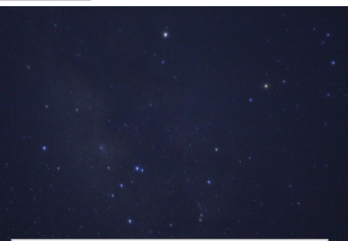
ライトダウン後の土星とさそり座
